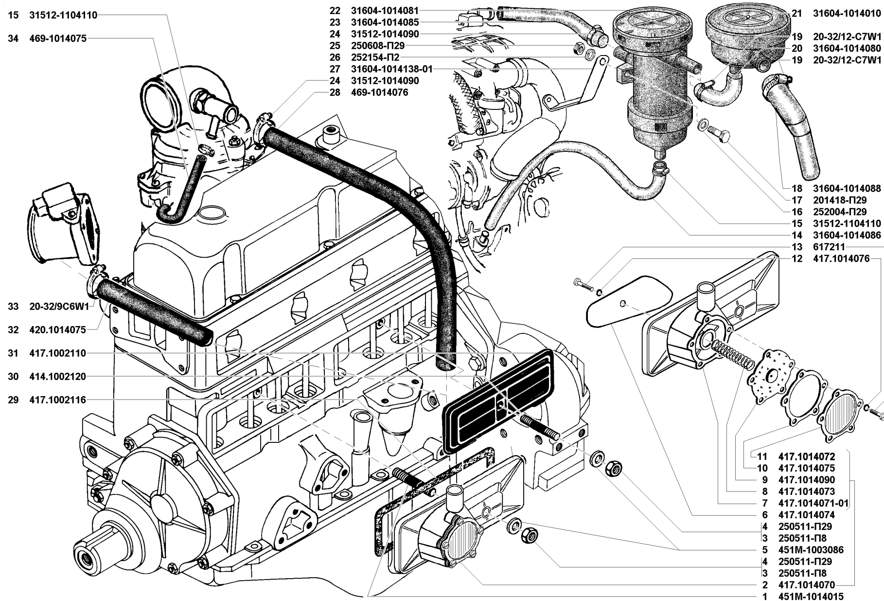
Рис. 14. Вентиляция картера (1014)
